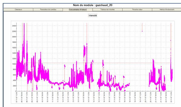
Suivi de la concentration d'odeurs en uoE/m 3
