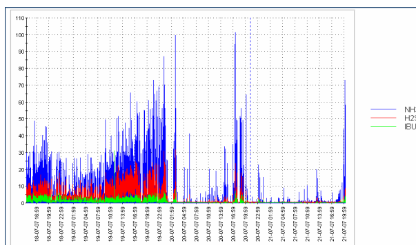
Suivi de la concentration en gaz cibles (ici H 2 S, NH 3 , COV) en ppm
